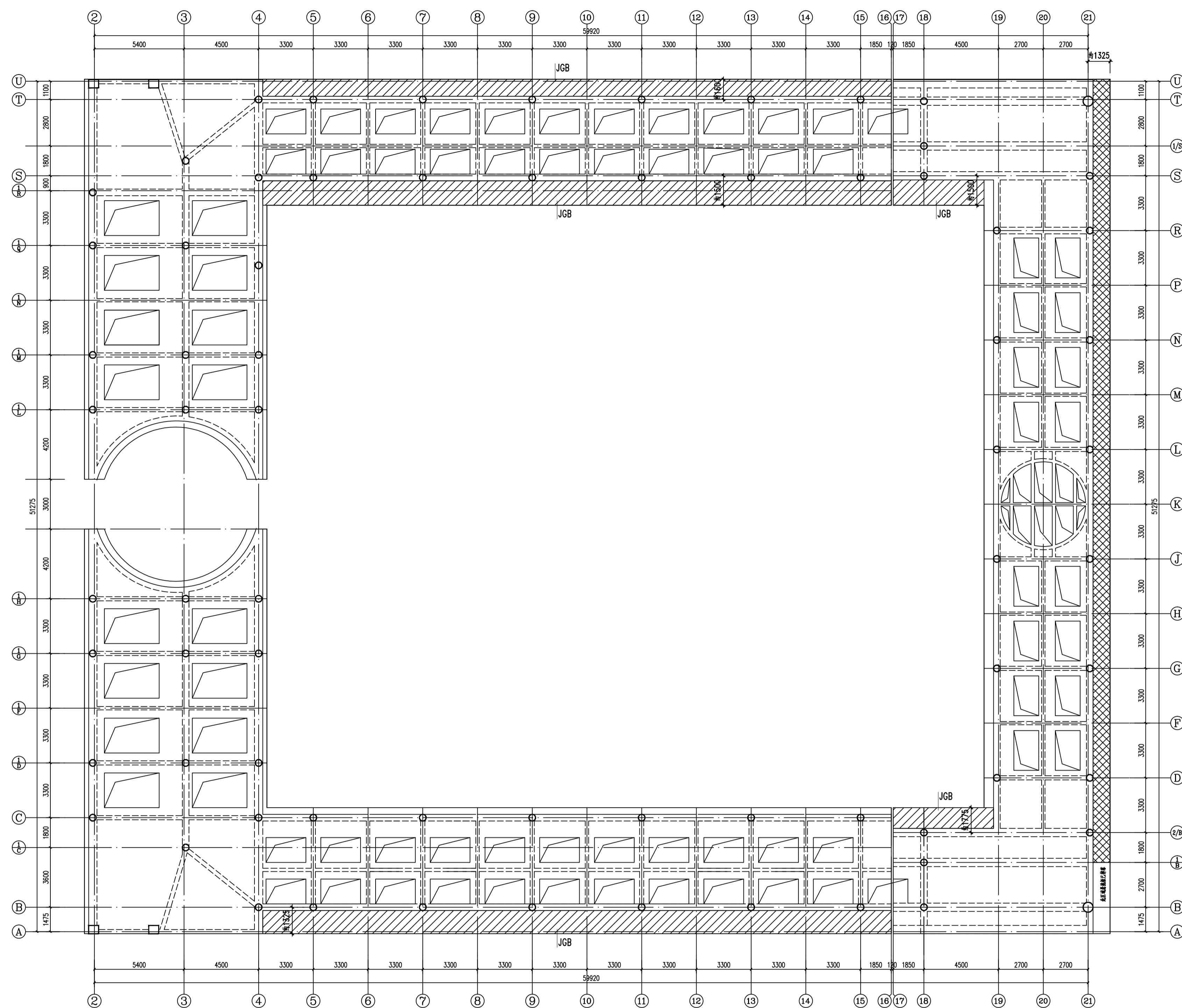
学生公寓厚德苑4号屋顶造型梁板加固平面布置图 1:150
