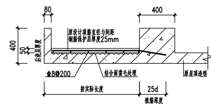
JGB大样图 1:25
